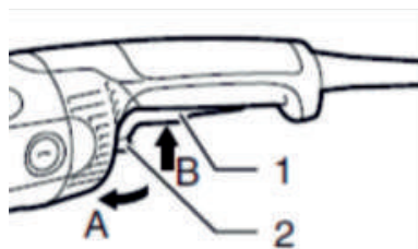
1 – курковый выключатель 2 – стопорный рычаг
